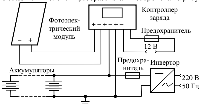
Рисунок 1 – Схема соединения блоков преобразователя
