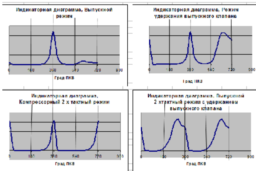
Рис. 3. Варианты индикаторных диаграмм в тормозном режиме
